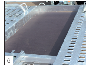
6 Serienausstattung: Multiplex- Zwischenboden zwischen den Fahrspuren auf der Vorderseite.
