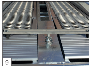
9 Serienausstattung: Befestigung der Auffahrampen zwischen den Fahrspuren.
