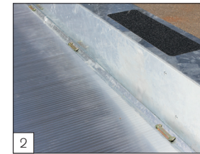
Serienausstattung: ausgestattet mit TÜV-geprüften Verzurrbügeln und Safety Steps an den Seiten.
