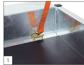
Serienausstattung: Verzurrbügel mit einer Kapazität von 1000 daN in den Boden integriert.
