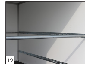
Option: Ladungssicherungssystem in dem geschlossenen Aufbau mit Sperrstange und Spanngurt.
