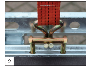
Standaard: voorzien van TÜV-goedgekeurde bindbeugels geïntegreerd in de zijrand, met een capaciteit van 1000 daN per stuk.
