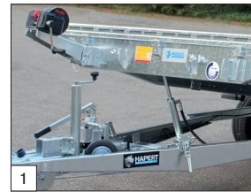
Standaard: met dubbelwerkend hydraulisch kipsysteem, en een vaste Combi Protect Rail 80 mm hoog, gemonteerd.
